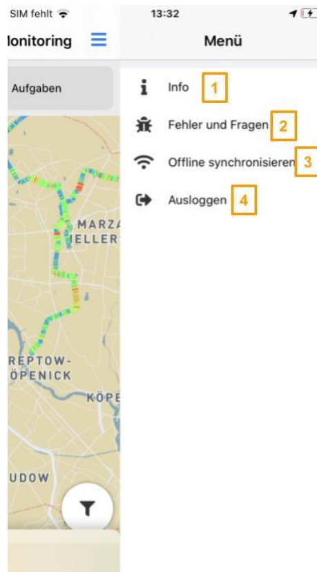
Abb. 2: Erweitertes Menü
