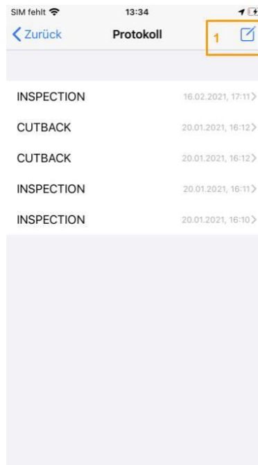
Abb. 8: Protokoll erstellen
