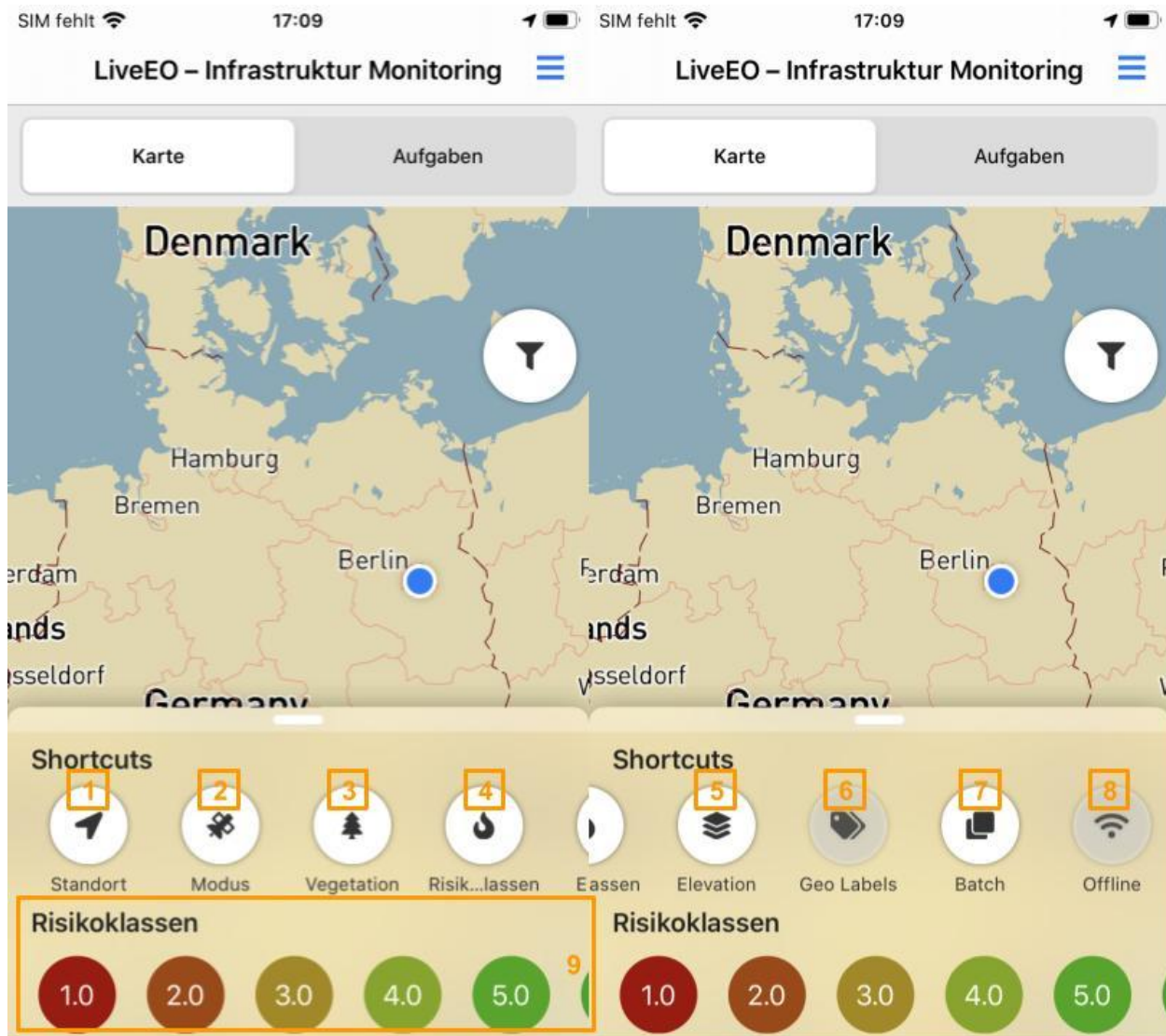
Abb. 4: Kontextmenü
